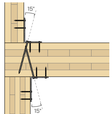
Beispiel: Montage der Winkelverbinder NINO15080 mit geneigten VGS-Schrauben zur Befestigung von Geschosswänden mit unterschiedlicher Stärke
