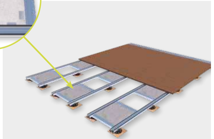
Windsogsicherung bei Holzterrassen mit Betonplatten und Auflastwinkel.
