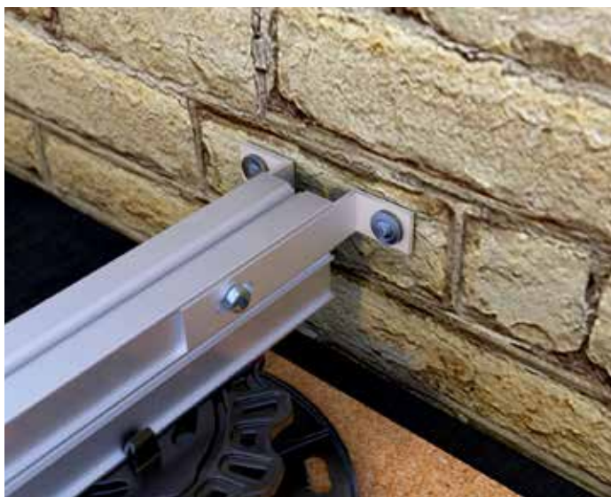
Anwendungsbeispiel Wandanschlusswinkel EVO
