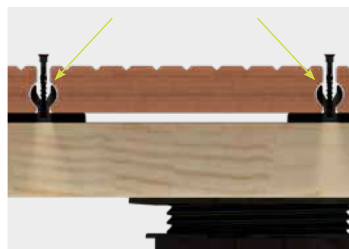
Der Kehlnutclip (K) auf einer Holzunterkonstruktion.*
