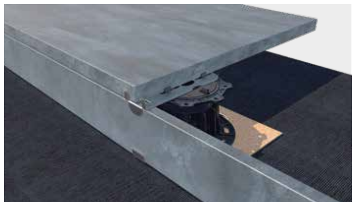
Einsetzen der Steinplatten in die Führungen der Randabschluss Einzelauflagerung.
