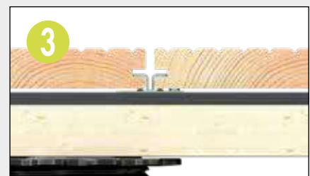
Befestigung der Bretter mit einer Spannzwinde, bis die Fuge des Holzes 5 mm beträgt.
