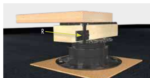
Befestigung einer Holzdielen auf einer Holzunterkonstruktion mithilfe des Rastverbinders (R).
