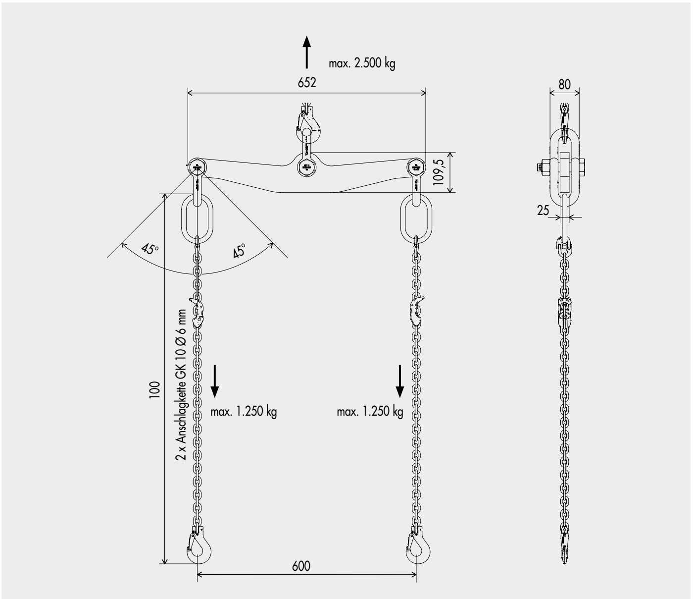
Anwendungsbeispiel mit Anschlagketten
